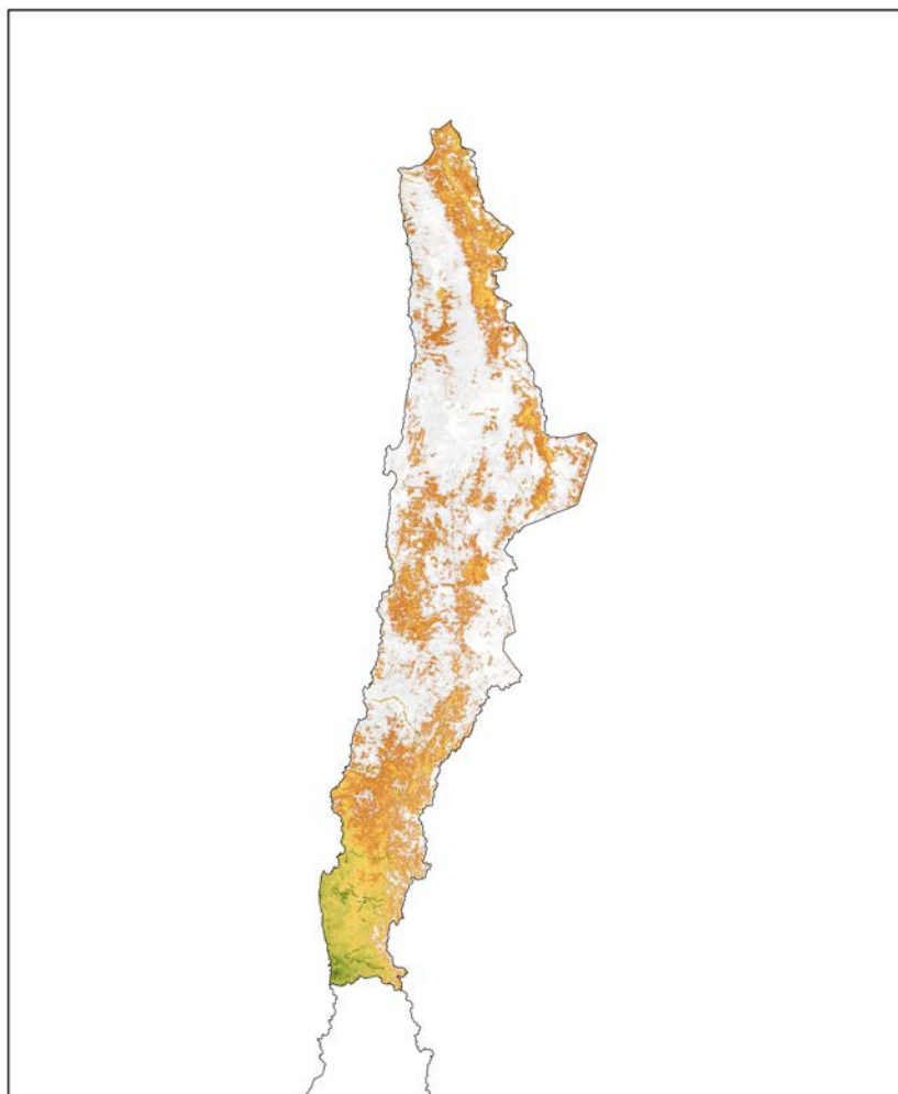
Figura 4.- Índice Normalizado de Vegetación NDVI de las macro zonas a) Norte Grande y Norte Chico.
